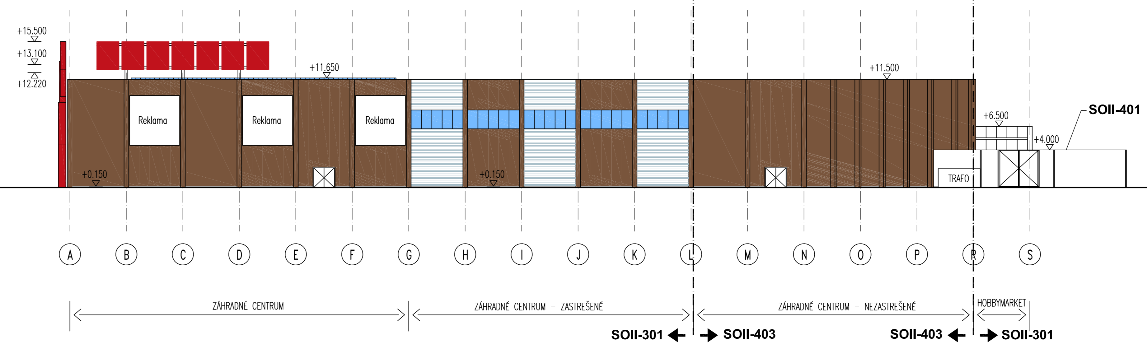
POHĽAD JUŽNÝ P 1:250
