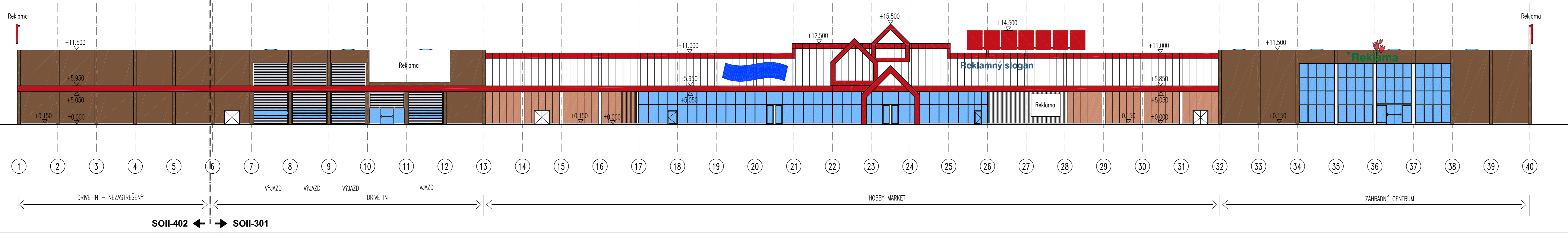
POHĽAD ZÁPADNÝ P 1:250
