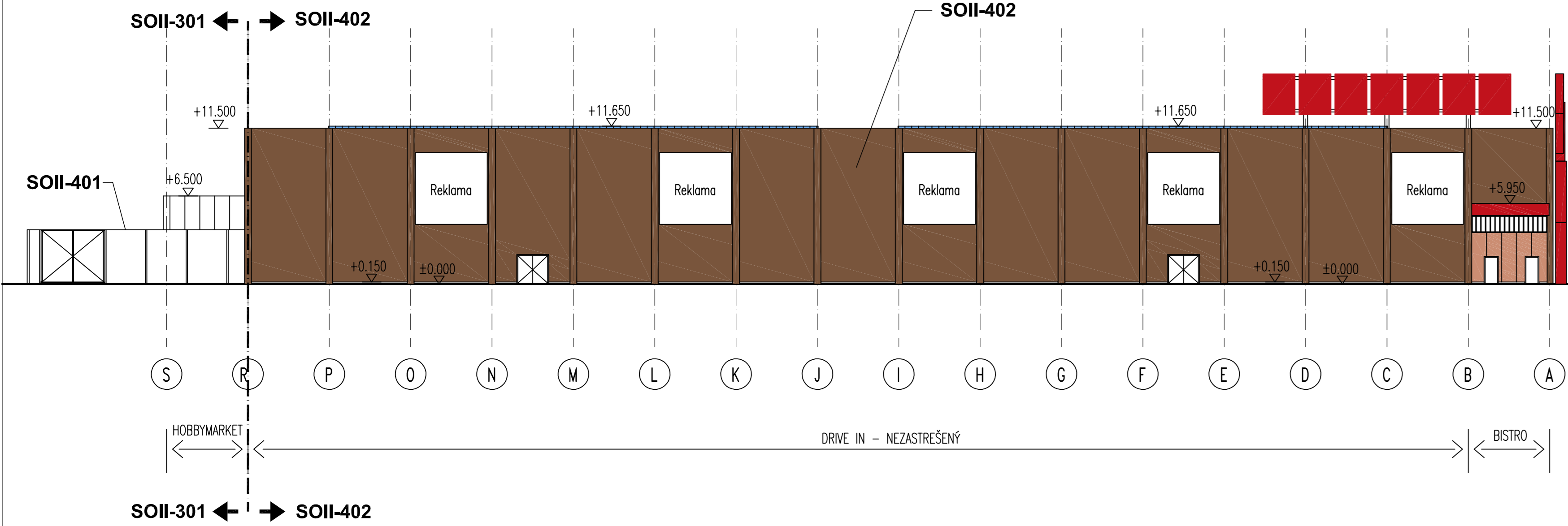
POHĽAD SEVERNÝ P 1:250
